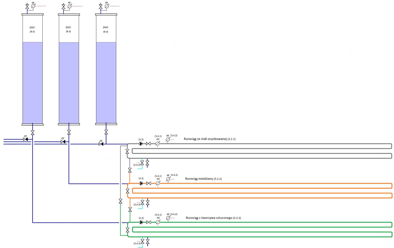
Rys.2 Schemat stanowiska dydaktyczno-badawczego do analizy systemu uzdatniania i dystrybucji wody przeznaczonej do spożycia - model sieci wodociągowej
