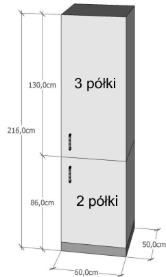
S9 - szafa gospodarcza 60x50 wys. 216cm obudowa, cokół - kolor c.szary drzwiczki - koloe szary
