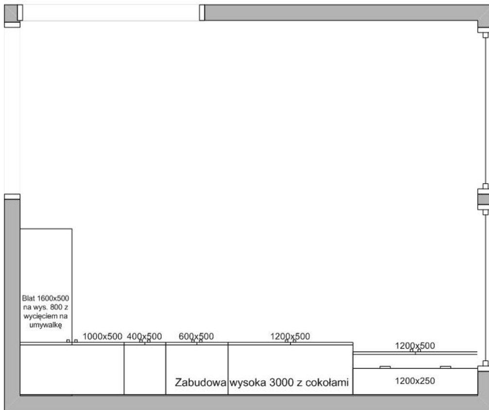
Rys. 2. rzut zabudowy
