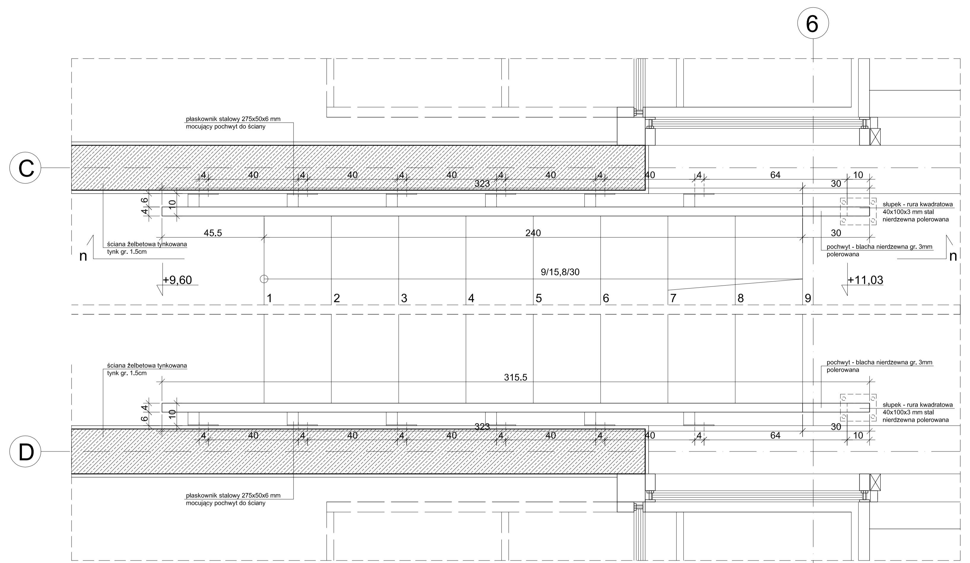
6 PRZEKRÓJ p - p
