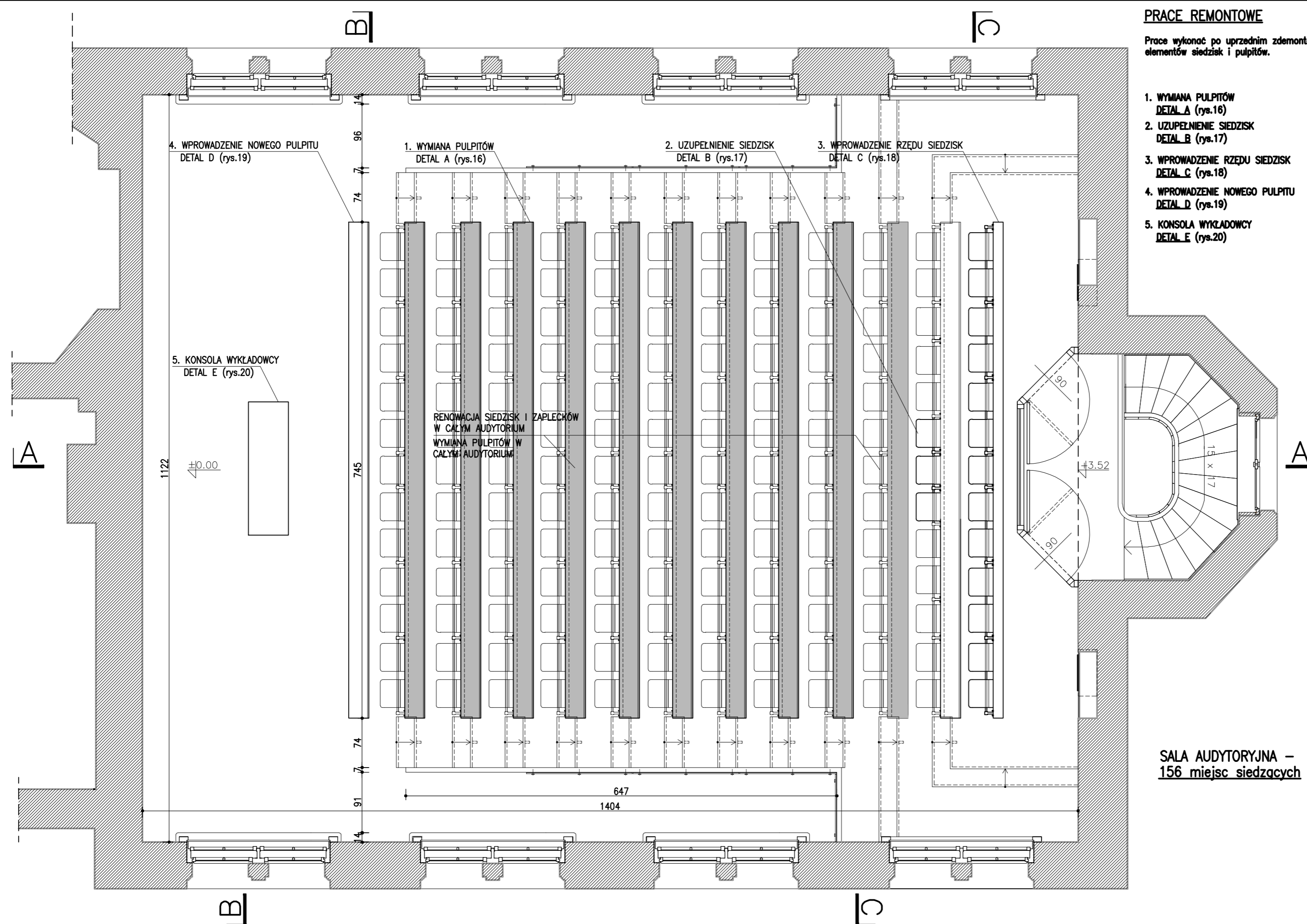
UMEBLOWANIE – RZUT NA WYSOKOŚCI ANTRESOLI 1:50
