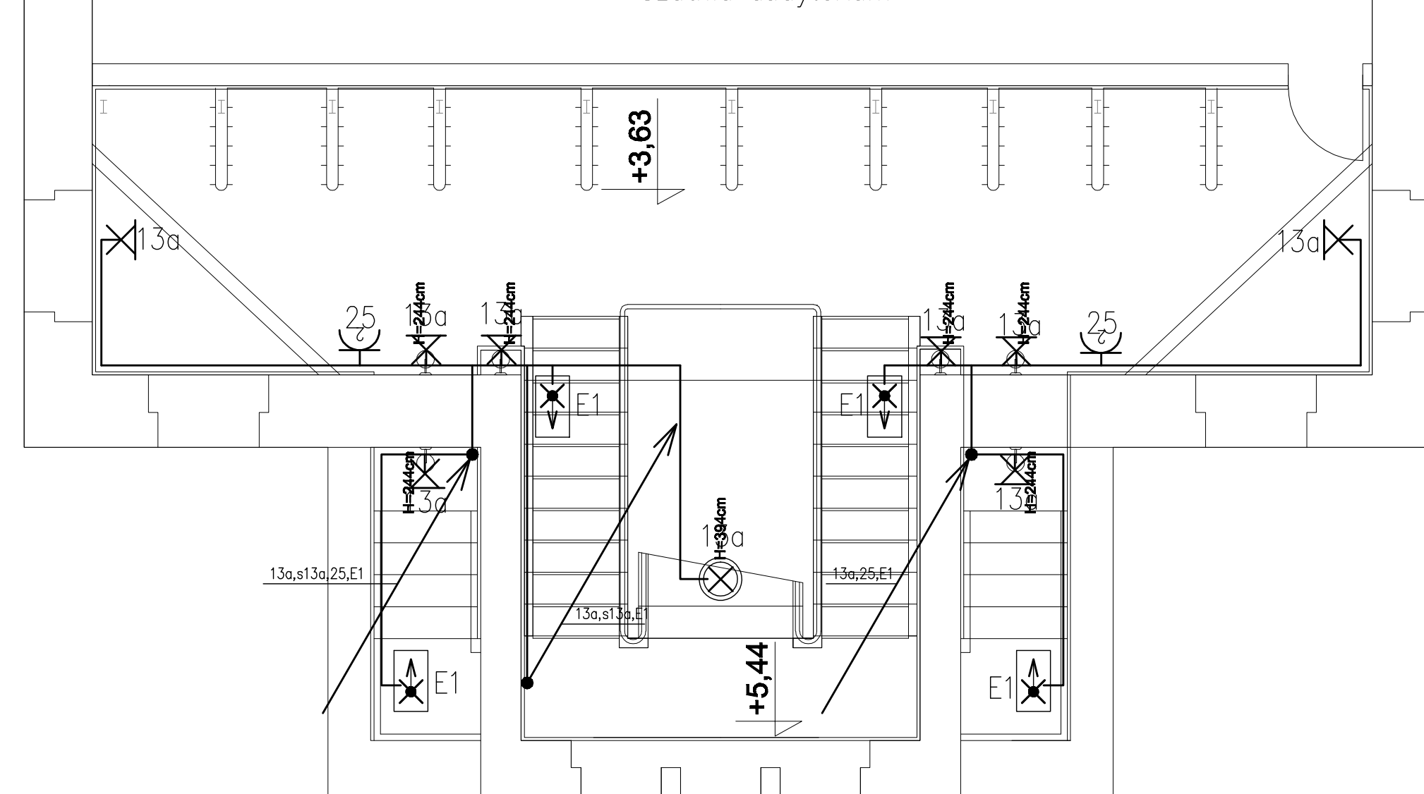
KLATKA SCHODOWA-PIĘTRO I (poz. +3.65)
