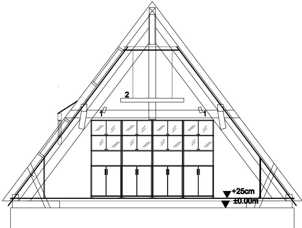
WIDOK ŚCIANY C 1 : 50
