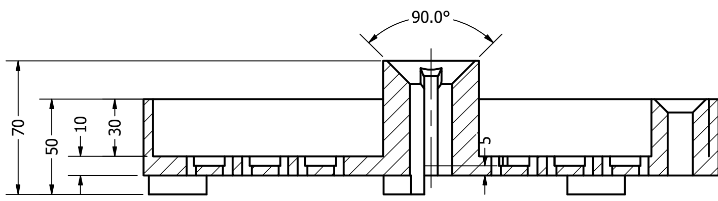
PRZEKRÓJ B-B SKALA 0,5
