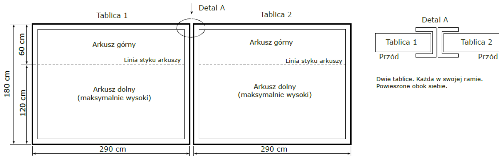
Rys. 2. Ułożenie tablic w miejscu montażu.
