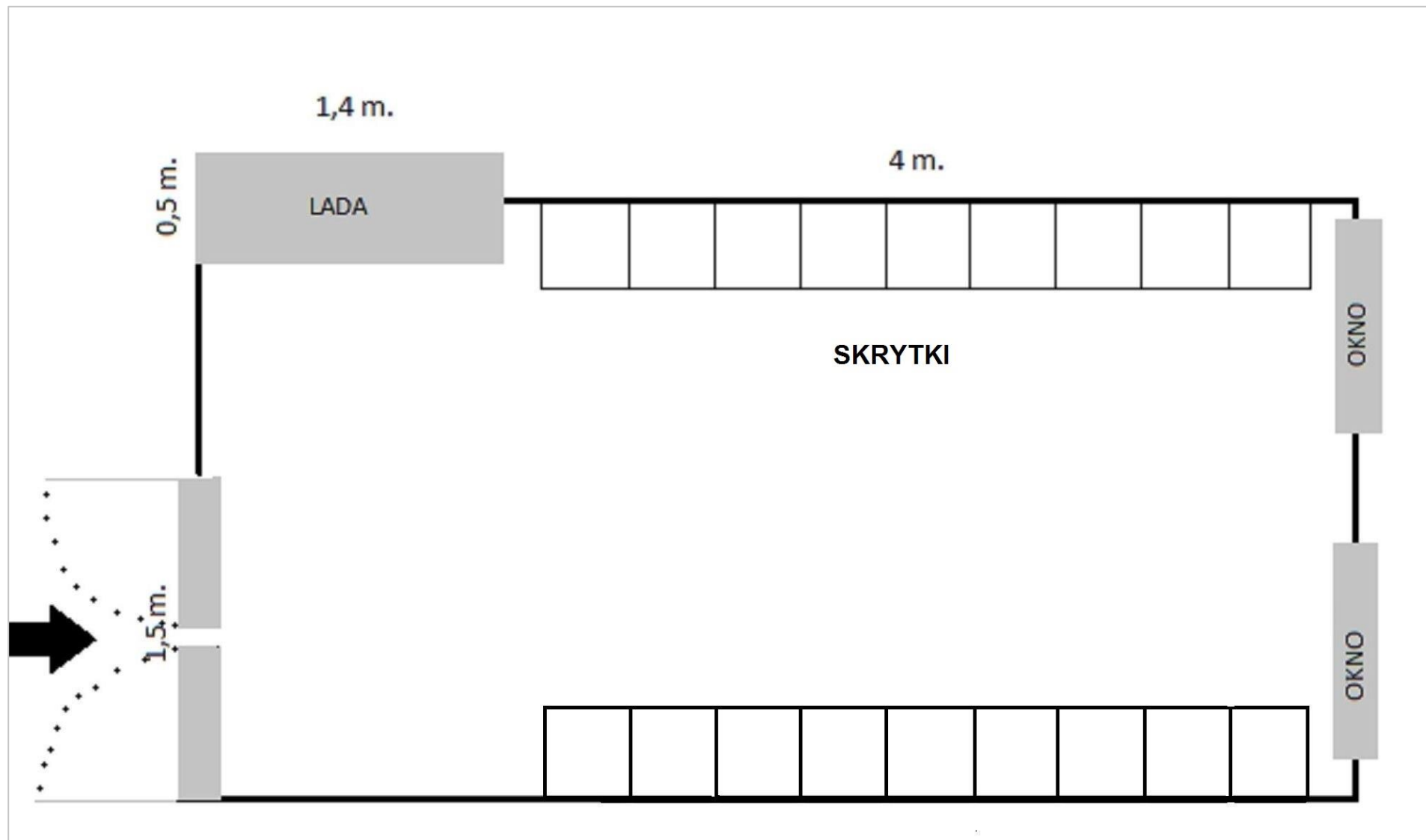
Rysunek nr 2a – skrytki pocztowe elektryczne z szufladami – widok z góry
