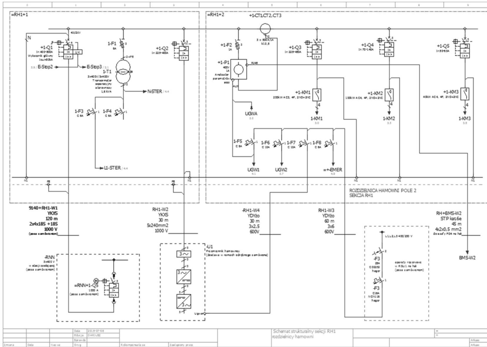
Rys. 1 Schemat strukturalny sekcji RH1 rozdzielnic hamowniczych
