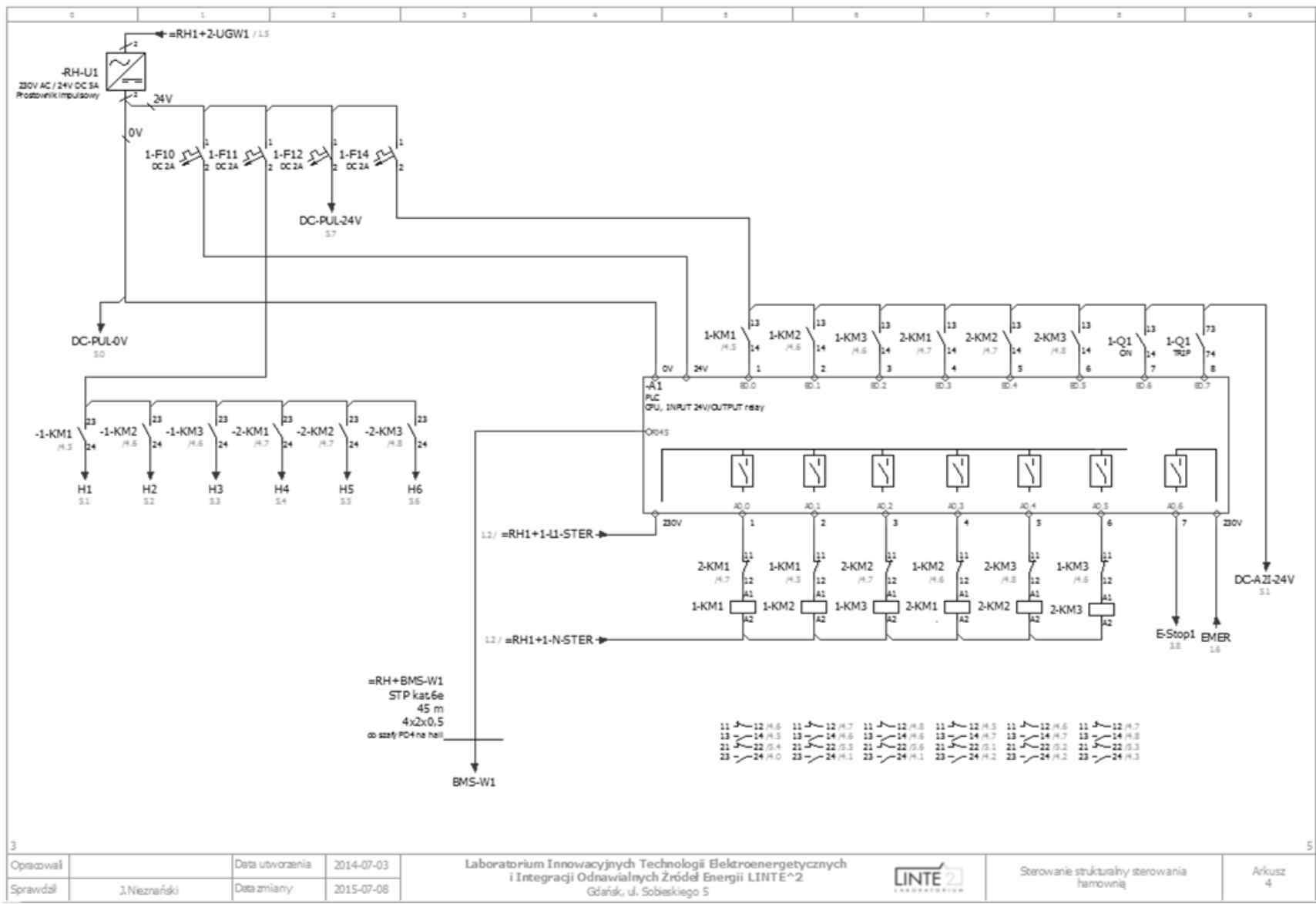
Rys. 4 Schemat strukturalny układu sterowania rozdzielnicy hamowni
