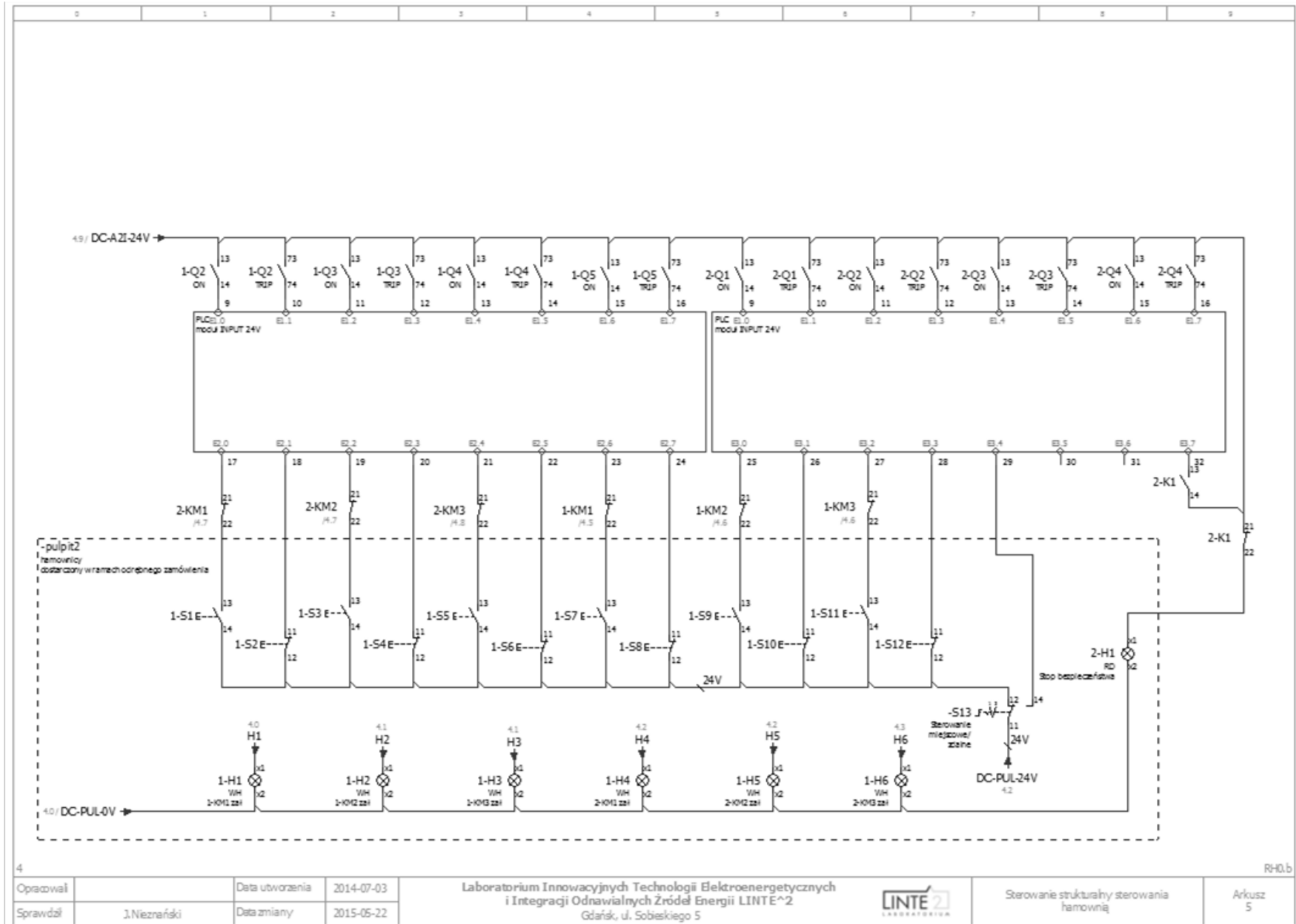
Rys. 5 Schemat strukturalny układu sterowania rozdzielnic hamowni (cd.)
