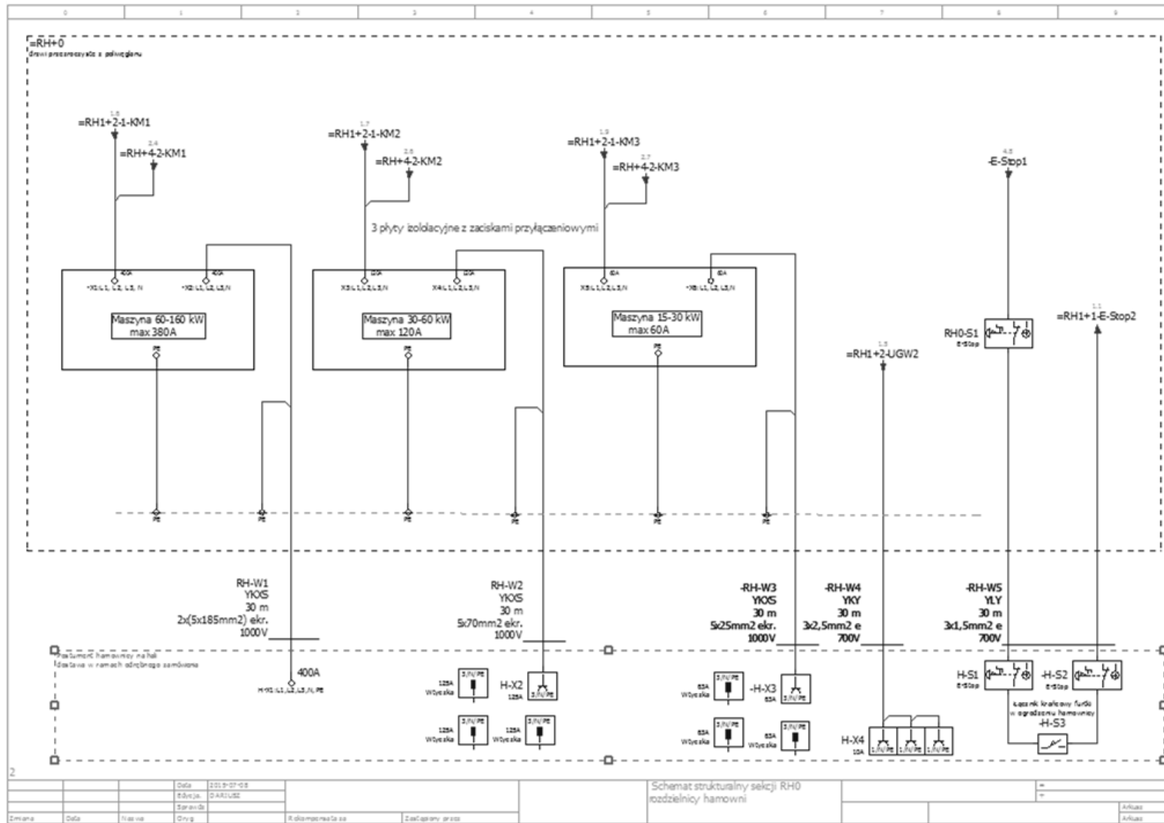
Rys. 3 Schemat strukturalny sekcji RH0 rozdzielni hamowni
