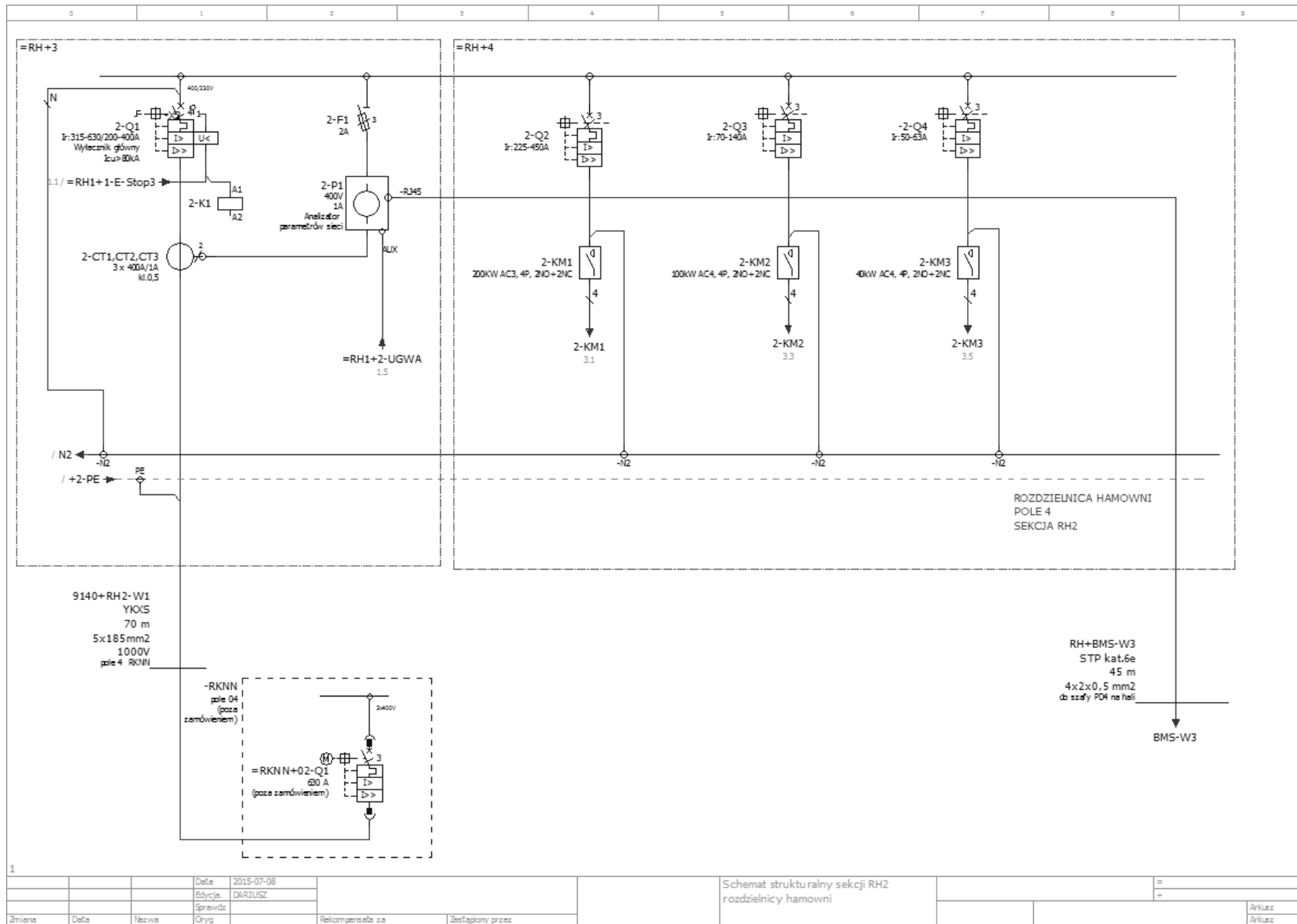
Rys. 2 Schemat strukturalny sekcji RH2 rozdzielnic hamowni
