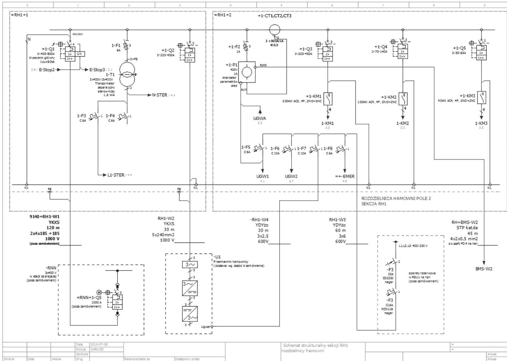
Rys. 1 Schemat strukturalny sekcji RH1 rozdzielnic hamowni
