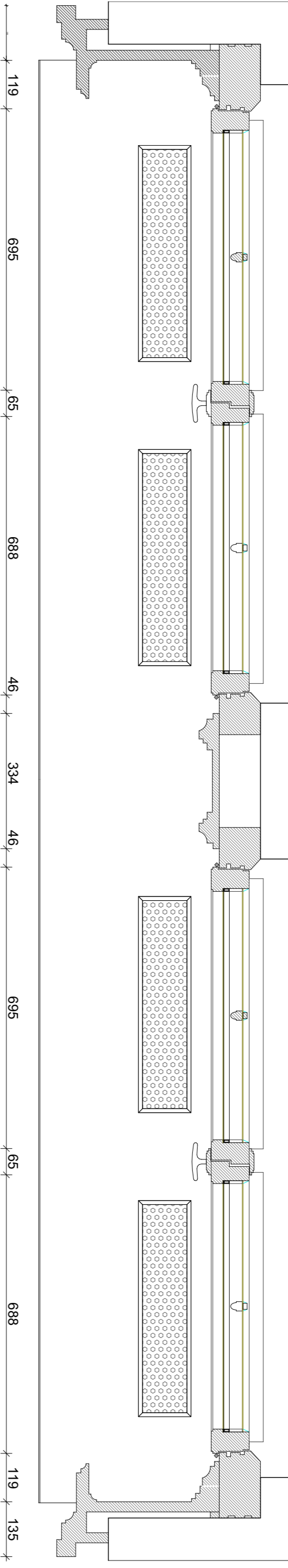
PRZERZĄCZ POZIOMY A-A - STAN ISTNIEJĄCY
