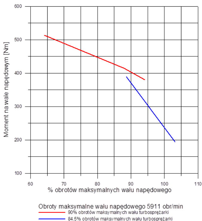
Rys. 1. Charakterystyka silnika GTD 350
