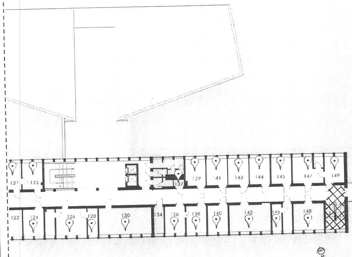
Rzut I piętra z zaznaczonym obszarem podlegającym remontowi Na piętrach od II do VII (obszar remontu jak na I piętrze)
