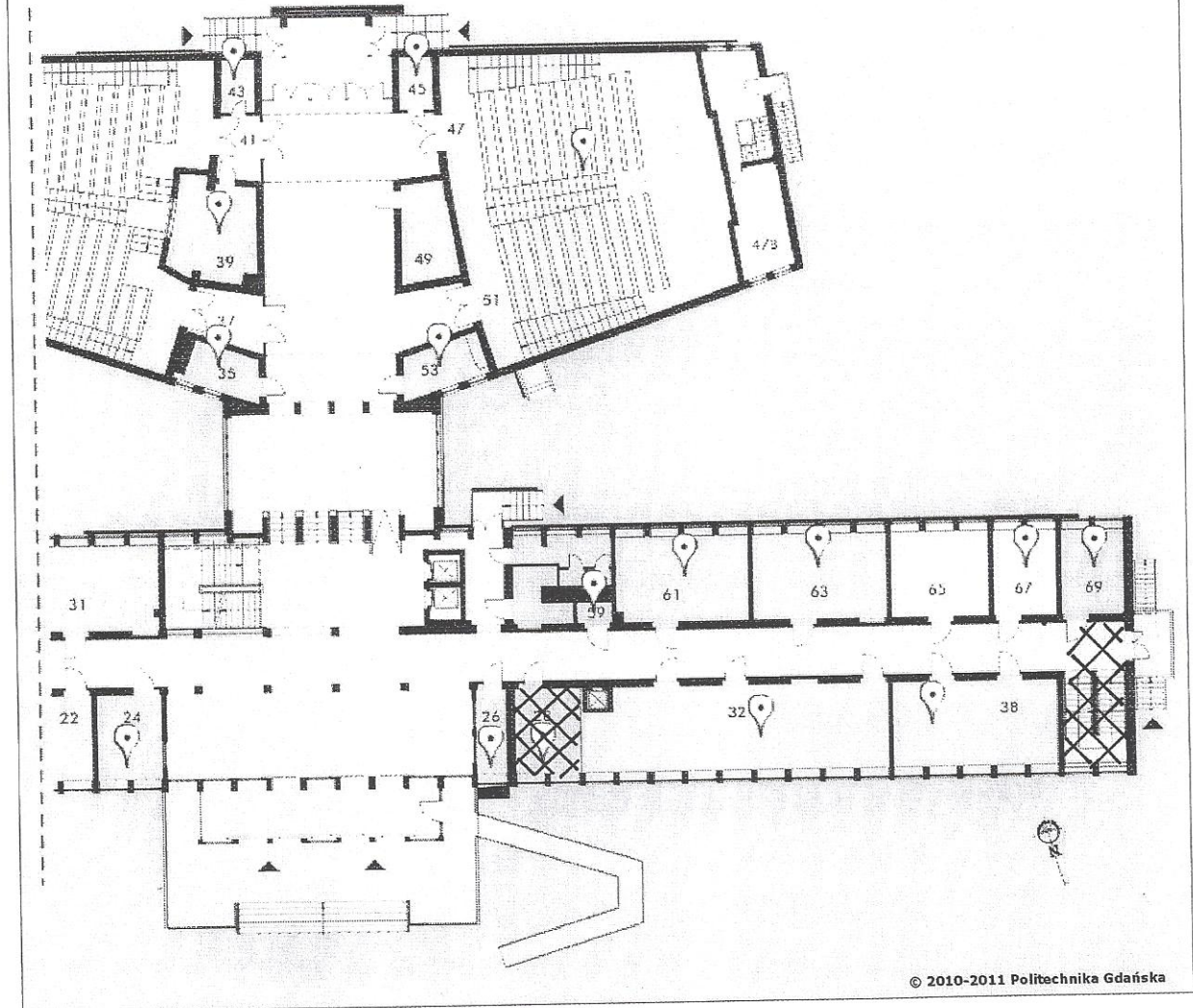
Rzut parteru z zaznaczonym obszarem podlegającym remontowi
