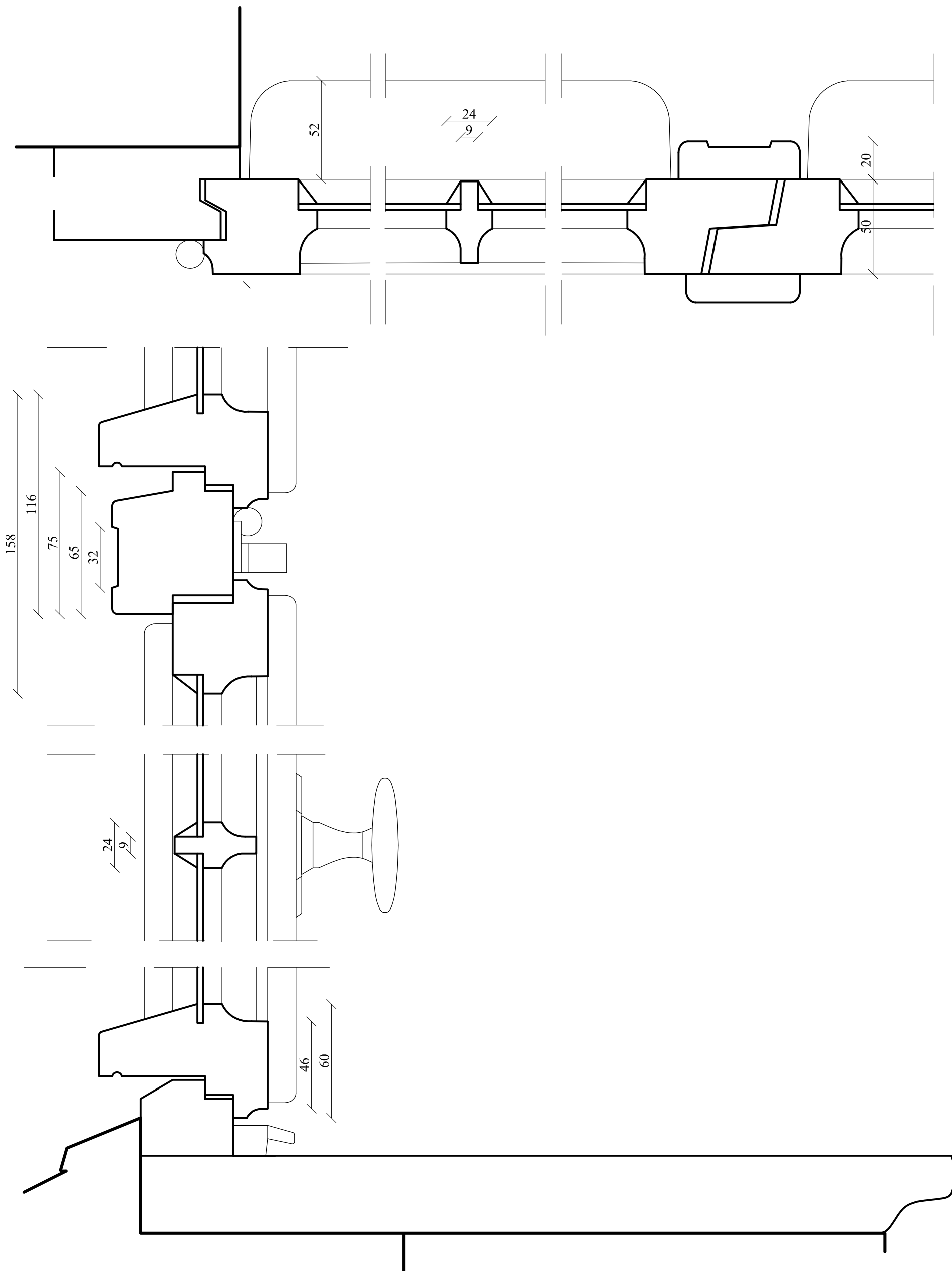
PRZEKROJE PRZEZ KONSTRUKCJĘ KROSNOWĄ OKNA ZABYTKOWEGO
