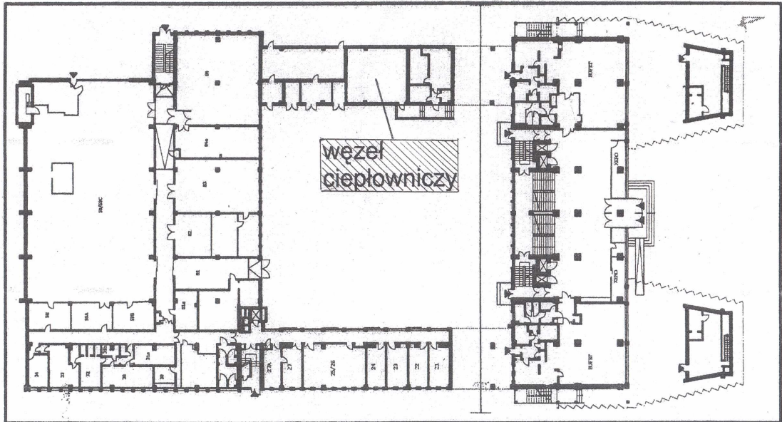
Rys. nr 1. Rzut parteru budynku WOiO Politechniki Gdańskiej.
