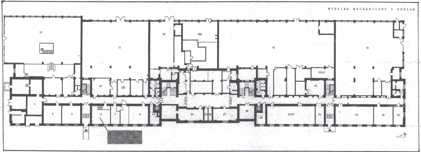
Rys. nr 3 Rzut parteru budynku Wydziału Mechanicznego Politechniki Gdańskiej.
