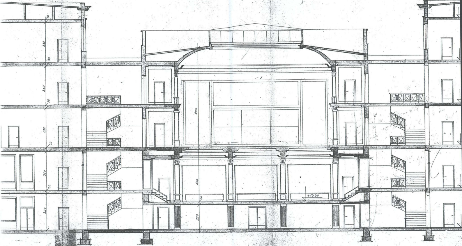
WYDZIAŁ MECHANICZNY PRZEKRÓJ
