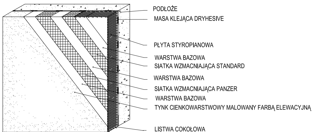
WZMOCNIENIE DODATKOWE
