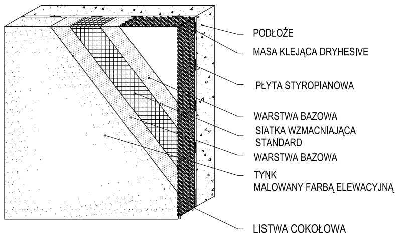
WZMOCNIENIE DODATKOWE
