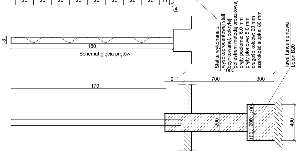
PRZEKRÓJ PRZEZ SŁUPEK
