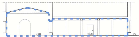
Przekrój A-A - Lokal Gastronomiczny Budynek Auditorium Maximum PG
