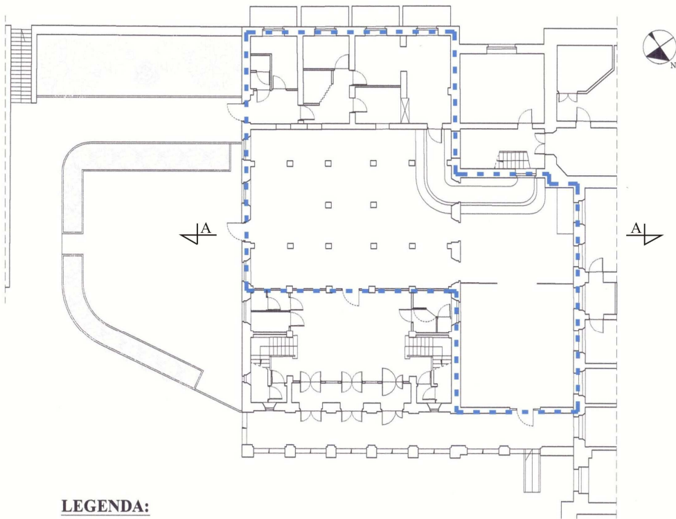
Rzut parteru - Lokal Gastronomiczny Budynek Auditorium Maximum PG
