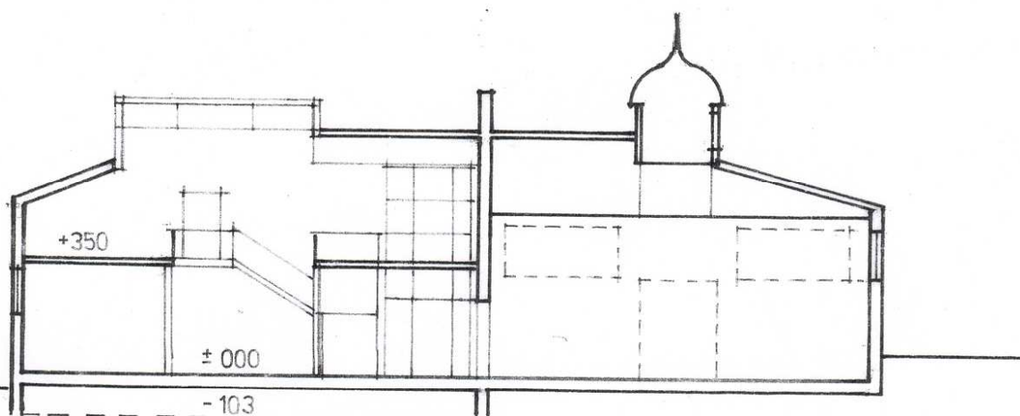
PRZEKRÓJ 1:200
