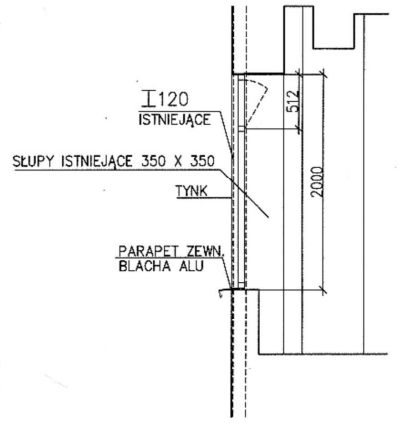
okno I piętro i II piętro A-A
