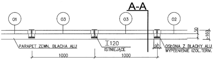
okna I piętro i II piętro
