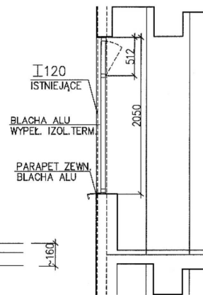
okno I piętro i II piętro A-A
